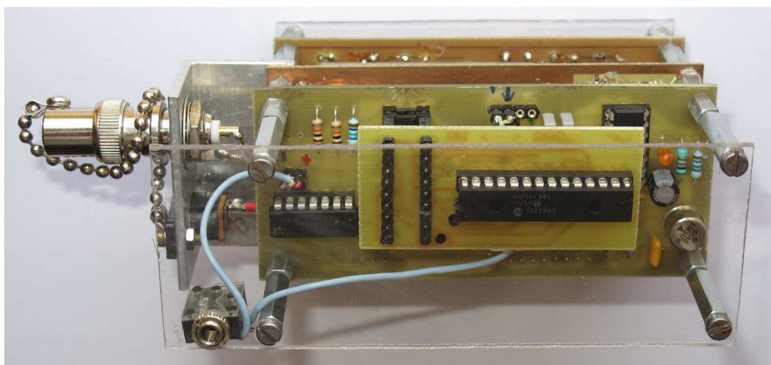
Photo 2 : La balise 406 : le PIC 16F886 fonctionne à la place du 16F88 par une carte d'adaptation
