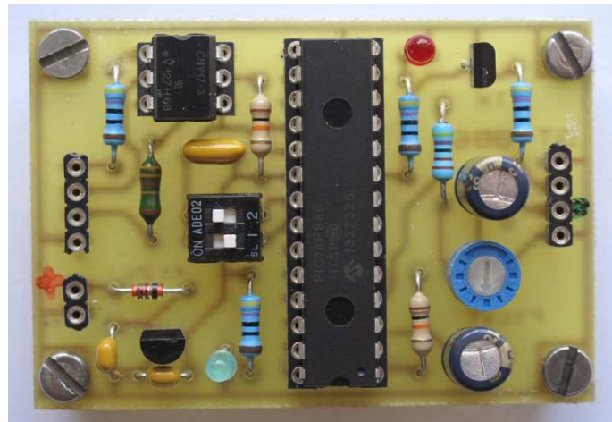
Photo 1 : Générateur de trames fonctionnant avec un PIC 16F886
