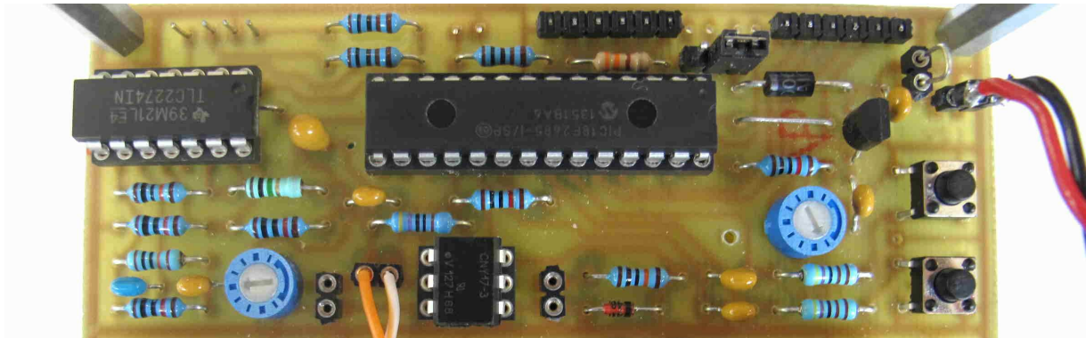
Photo 2 : Connexion du GPS sur la carte DECTRA. Les deux entrées GPS sont situées de part et d'autre du circuit CNY17-3.
