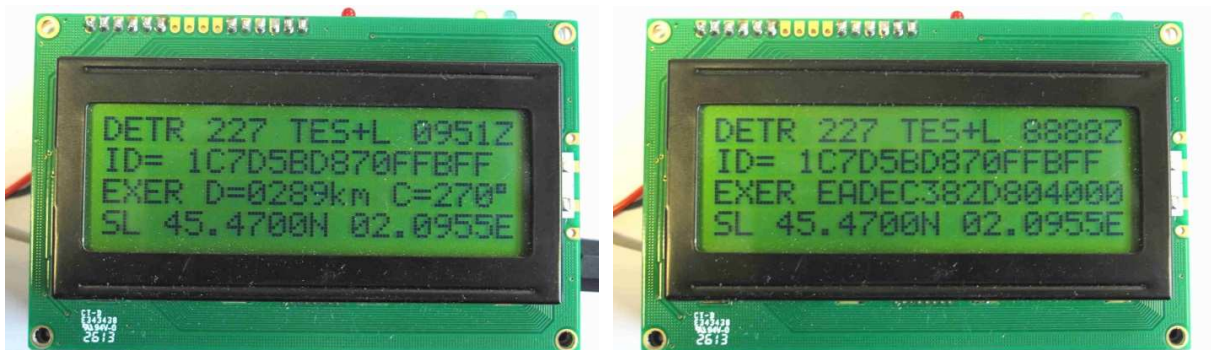
Photos 3 et 4 : Affichage de distance et du cap : - avec GPS connecté au décodeur - sans GPS connecté au décodeur
