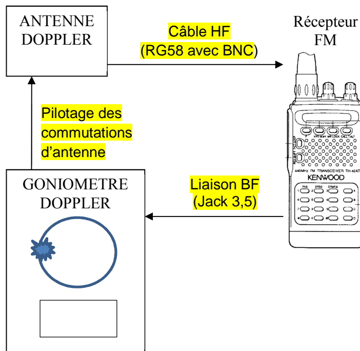
Figure 1 : Le radiogoniomètre Doppler complet avec ses 3 sous-ensembles : l'antenne Doppler, le récepteur FM, et le boîtier de pilotage et d'affichage. Pour relier ces 3 sous-ensembles, il faut 3 câbles : le câble HF (5m de RG58 avec prises BNC), la liaison BF (avec un Jack 3,5 à chaque extrémité) et le câble de transmission des signaux de commutation.
