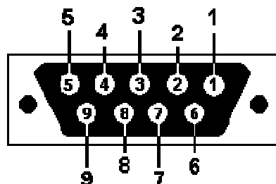
Figure 2 : Brochage de la prise DB9 femelle du boîtier Doppler
